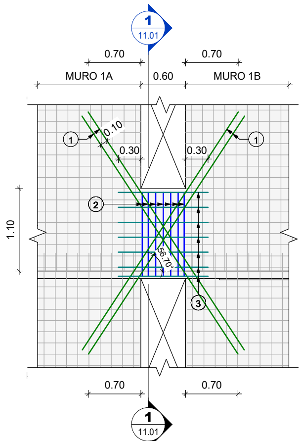
DETALLE 1 - VIGA DE ACOPLE Escala 1 : 50
