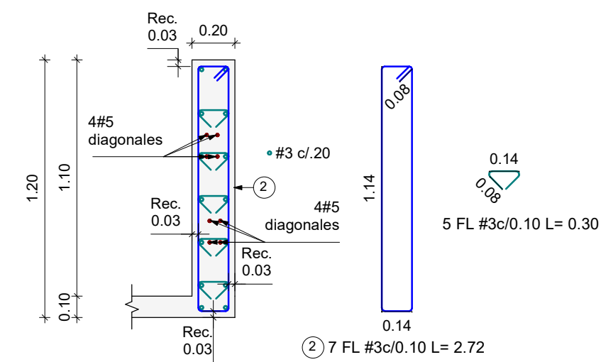
CORTE 1 - 1 VIGA DE ACOPLE TIPO 1 e=0.20 Escala 1 : 25
