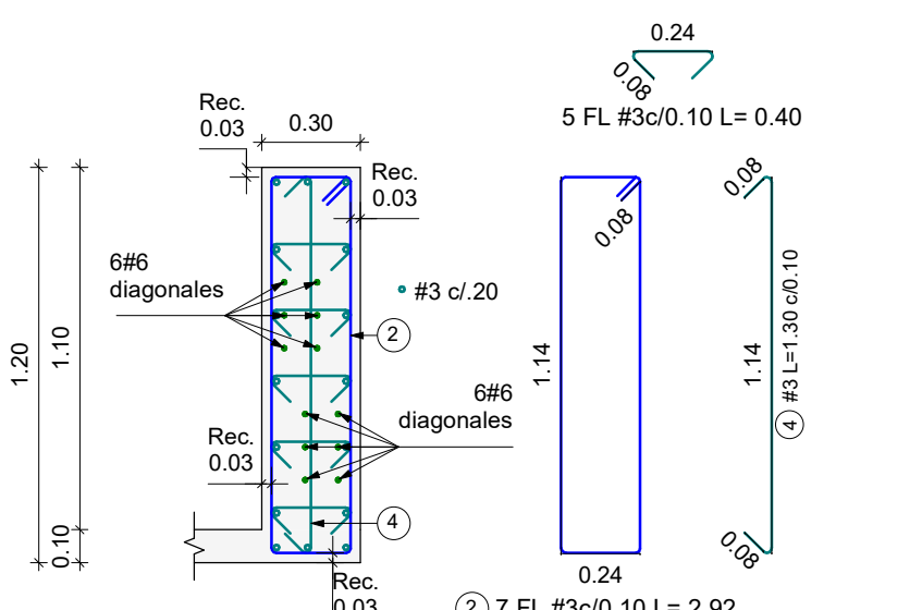
CORTE 2 - 2 VIGA DE ACOPLE TIPO 3 e=0.30 Escala 1 : 25
