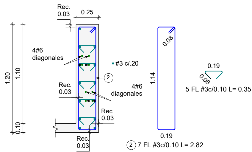
CORTE 1 - 1 VIGA DE ACOPLE TIPO 2 e=0.25 Escala 1 : 25
