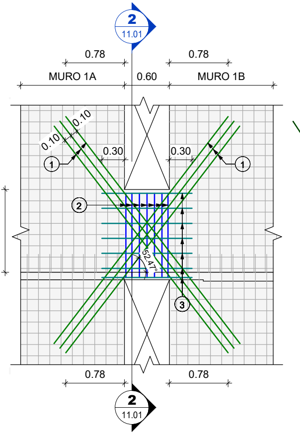
DETALLE 2 - VIGA DE ACOPLE Escala 1 : 50
